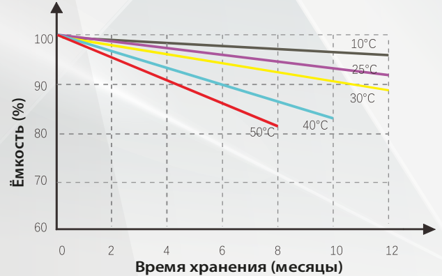
Саморазряд при хранении
