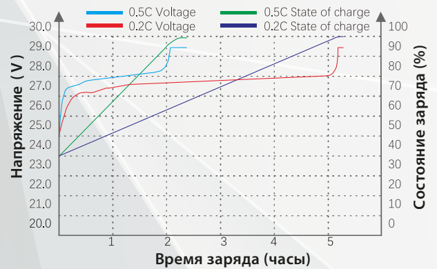
Кривая состояния заряда при 25°C
