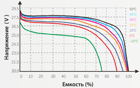
Разряд при различной температуре при 0.5C
